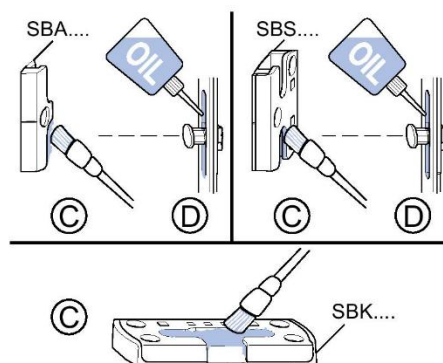
Smeerpunten
